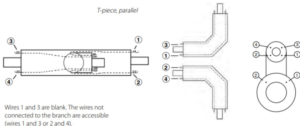
Figur 1 Alarmtegning for kobling av en parallellavgrening
